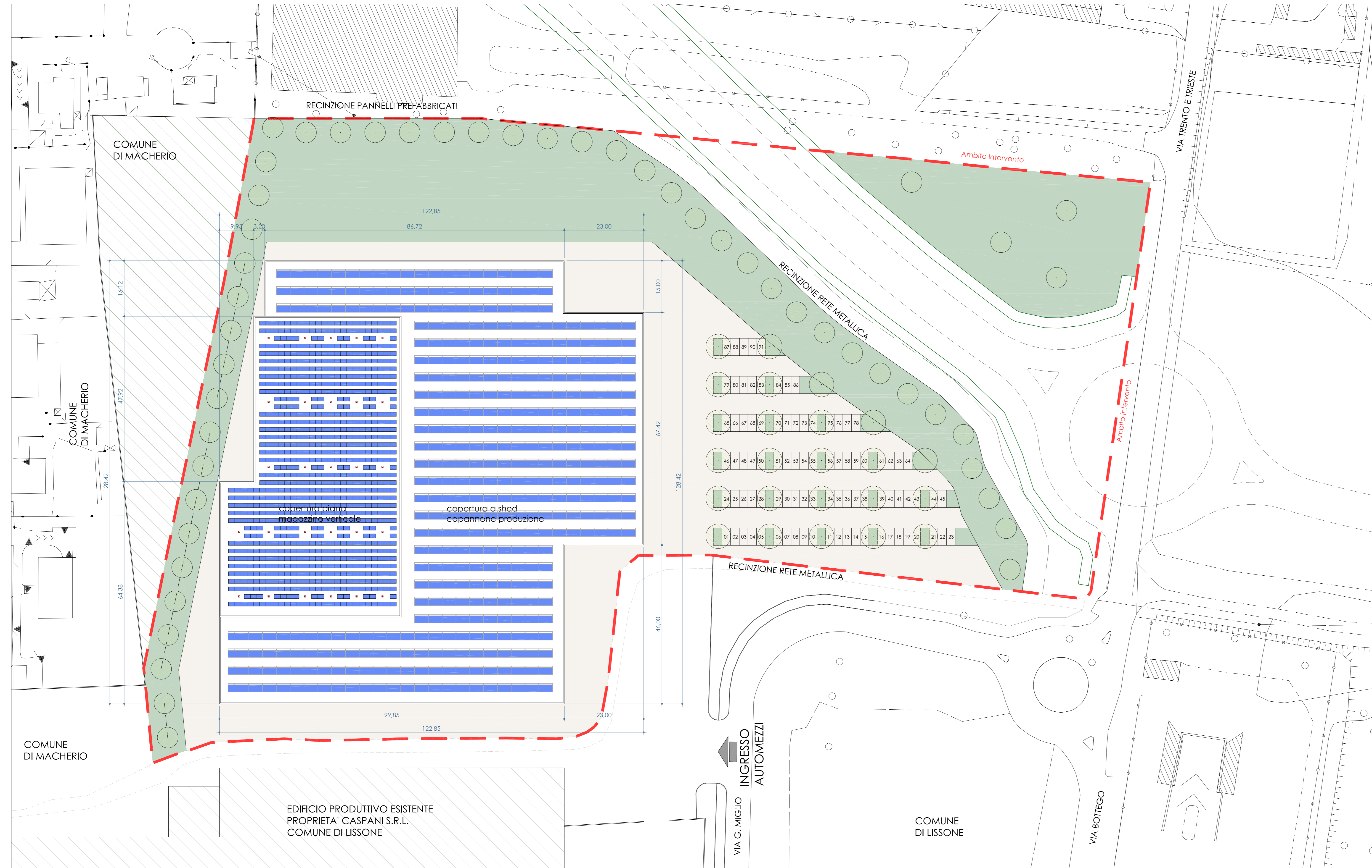
PLANIMETRIA GENERALE IN PROGETTO PIANTA COPERTURA
